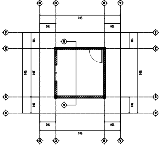
DENAH RENCANA SKALA 1 : 100
