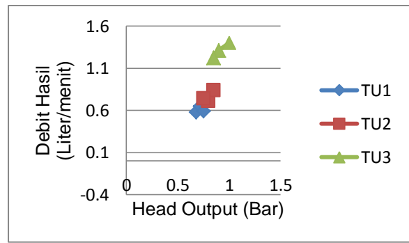
Gambar 1. Grafik Hubungan Antara Head Output dengan Debit Hasil Pada Berbagai Variasi Ukuran Tabung Udara
