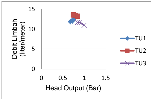
Gambar 2. Grafik Hubungan Antara Head Output dengan Debit Limbah Pada Berbagai Variasi Ukuran Tabung Udara
