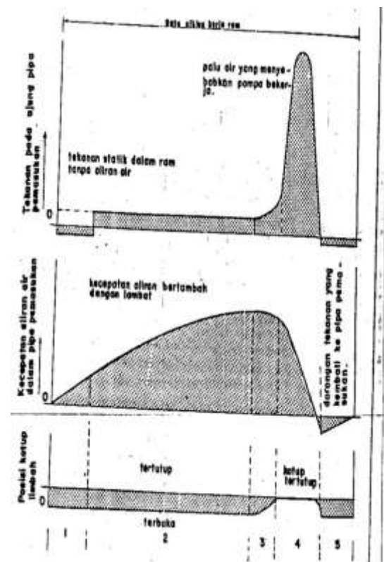
Gambar 2 diagram satu siklus kerja pompa hidram.
