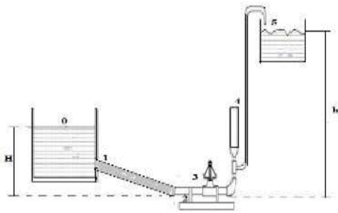
Gambar 3. Skema Instalasi Pompa Hidram
