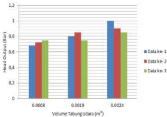
Gambar 4. Grafik Hubungan Antara Volume Tabung Udara dengan Head Output Pompa Hidram
