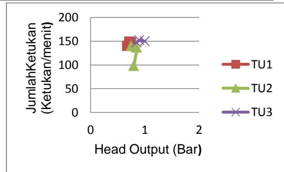
Gambar 3. Grafik Hubungan Antara Head Output dengan Jumlah Ketukan Katup Limbah Pada Berbagai Variasi Ukuran Tabung Udara
