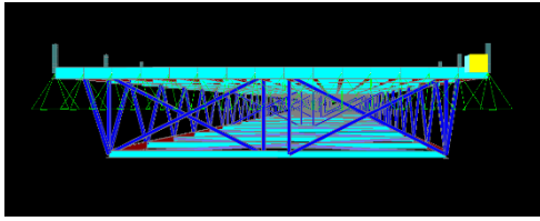
Gambar Gelagar Sap2000 arah YZ
